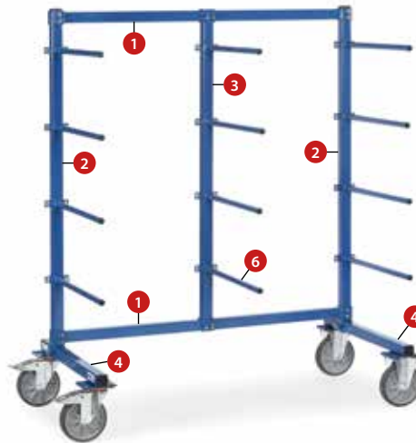
Komponenten für Tragarmwagen
