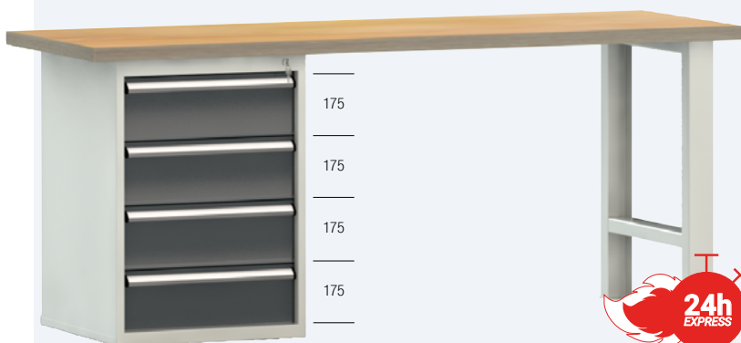
Standard-Werkbank WS515N-2000M40-E0804
